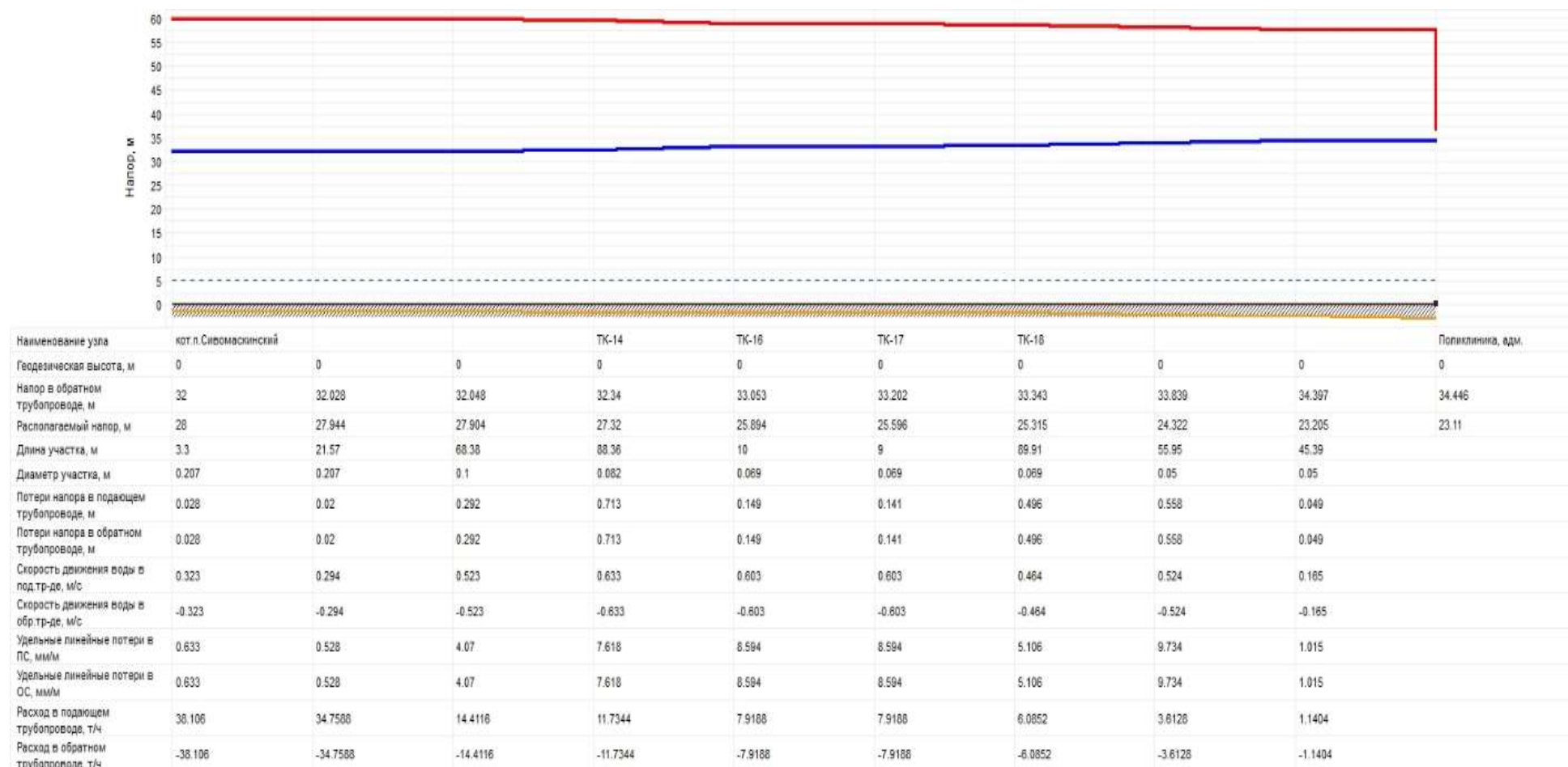
Рисунок 1.10 Пьезометрический график тепловых сетей пст. Сивомаскинский
