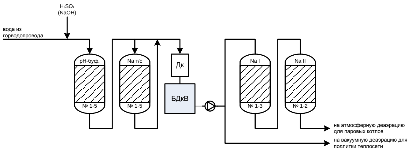
Рисунок 1.11. Принципиальная схема ВПУ
