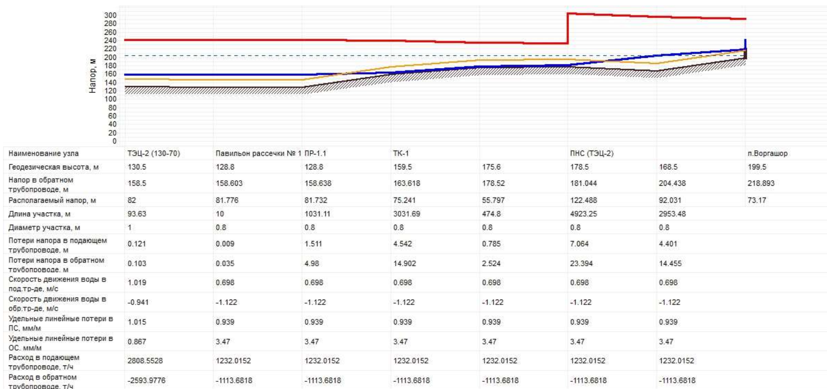
Рисунок 1.7 Пьезометрический график ТЭЦ-2 по тепловыводу «Запад»
