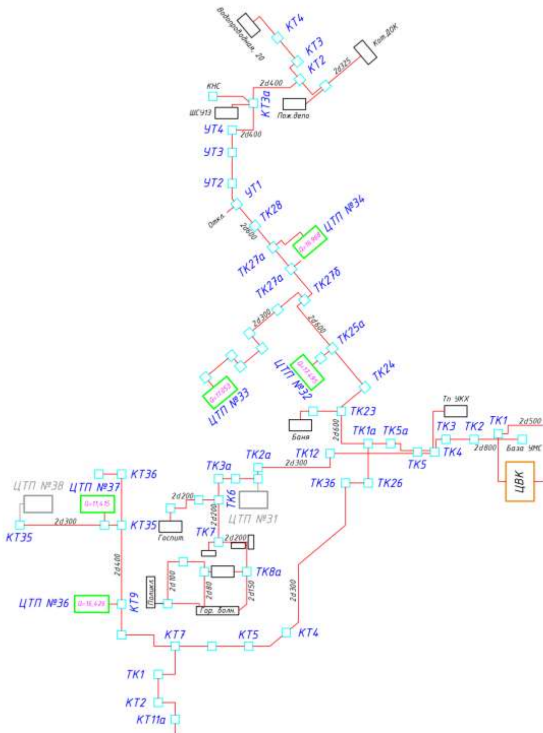
Схема теплоснабжения, г.Воркута от ЦБК Шахтерский район
